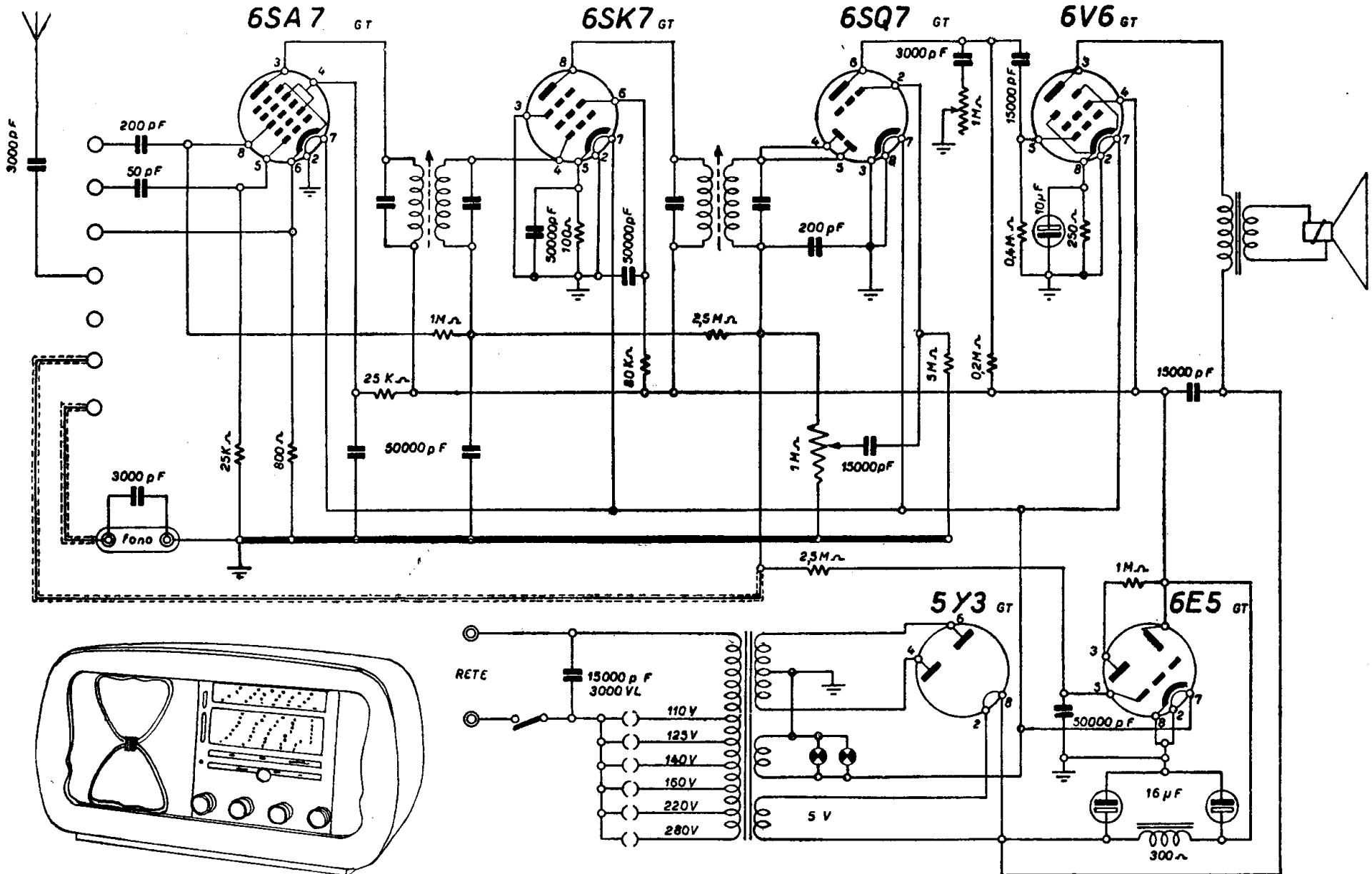
REOM - Sintomagic Radio mod. n2 - Ricevitore a quattro gamme d'onda. Media frequenza a 470 kc. Ochio magico. Controllo di tonalità. Resa d'uscita 4 watt. Consumo 60 watt.
